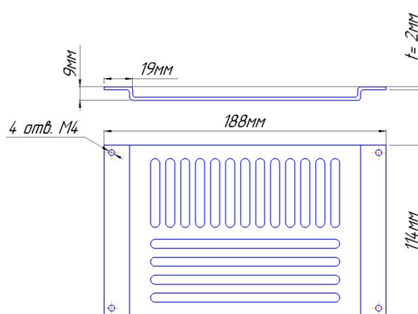
Чертеж 1. Габаритные размеры Н0-ZA1
