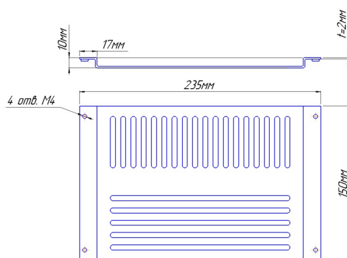
Чертеж 2. Габаритные размеры Н0-ЗА2
